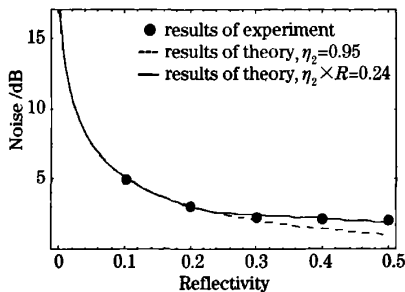
图4 剩余强度噪声与反射率的关系图
