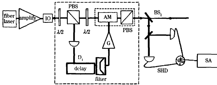
图 1 利用光电前置反馈方法抑制光纤激光器强度噪声的实验装置图
