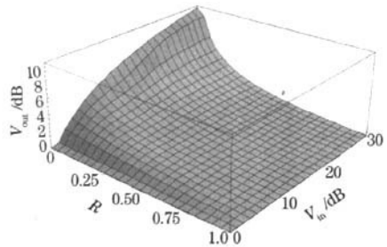
图3 最佳输出噪声 V_{out} 随输入噪声 V_{in} 和分束器的反射率 R 的变化关系。 \eta_2=0.95, \eta_3=0.20
