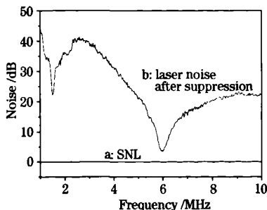
图5 在 6.0 MHz 处光电反馈的强度噪声的最佳抑制
