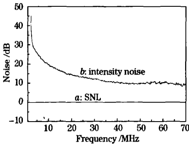
图 2 光纤激光器在 1~70 MHz 的强度噪声
